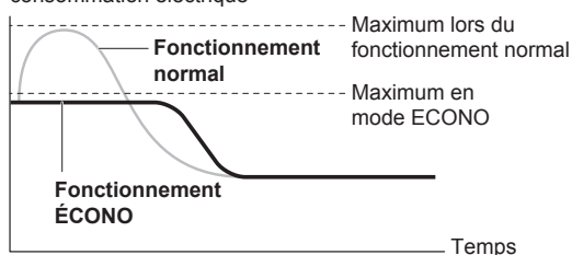
Courant de fonctionnement et consommation électrique
